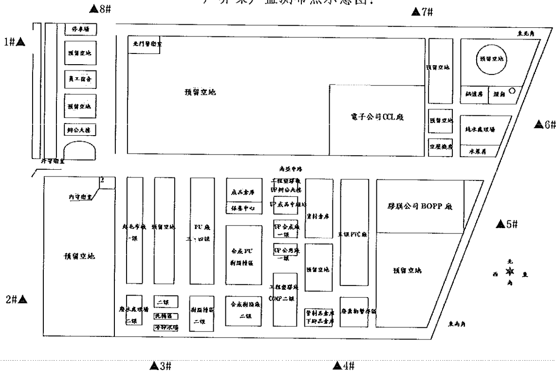
厂界噪声监测布点示意图:
