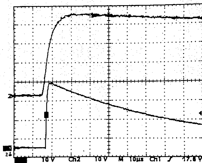
示波图
