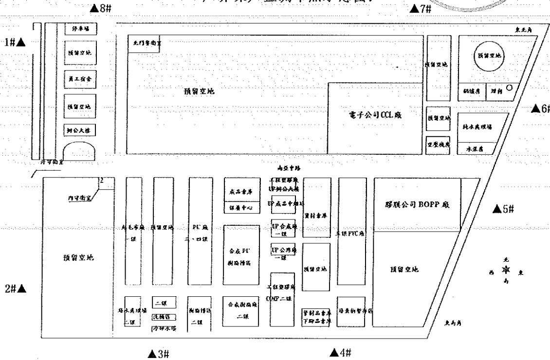
厂界噪声监测布点示意图:
